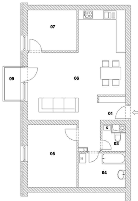
I. EMELET "A" 1/3 LAKÁS
