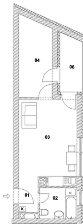
I. EMELET "B" 1/3 LAKÁS
