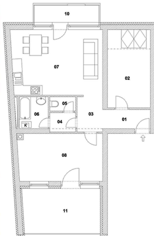
TETŐTÉR "A" 3/1 LAKÁS
